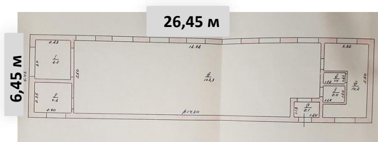
Будівля складу-ангару №2, 170,6 м 2
